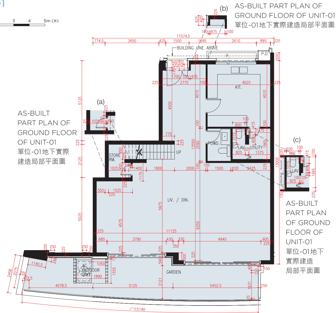
GROUND FLOOR PLAN 地下層平面圖
