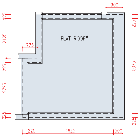
TOP ROOF PLAN 頂層天台平面圖
